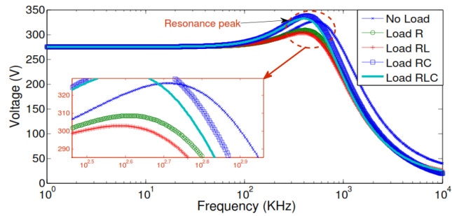
(b). LLCL+damper
