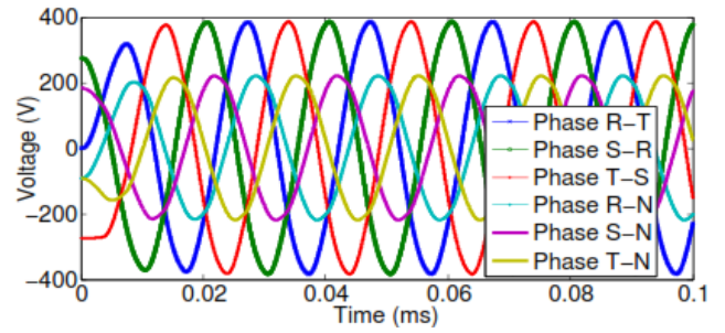
(a). LLCL+damper
