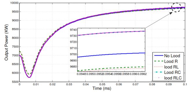
(a). LCL+damper
