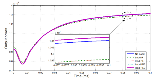
(d). LCL 3-leg
