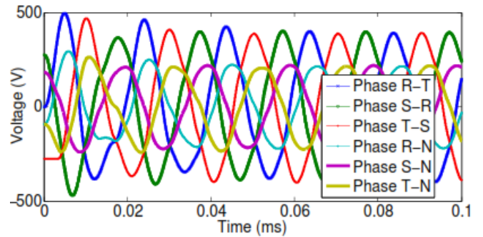
(b). LLCL+damper
